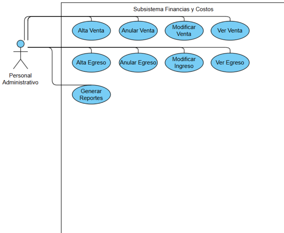
Figura 4 - Diagrama Caso Usos Subsistema Finanzas y Costos
