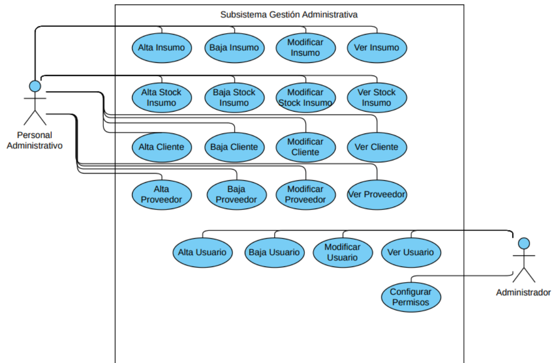
Figura 5 - Diagrama Caso Usos Subsistema Gestión Administrativa
