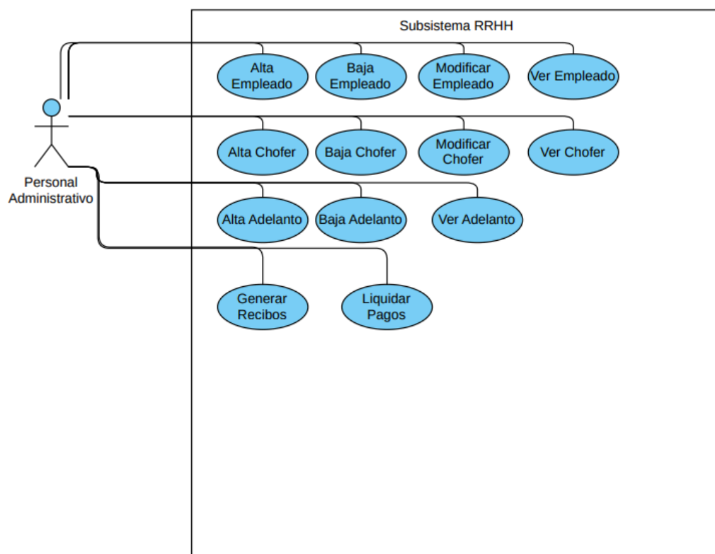
Figura 3 - Diagrama Caso Usos Subsistema Recursos Humanos
