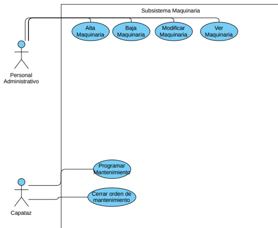
Figura 2 - Diagrama Caso Usos Subsistema Maquinaria y Equipos
