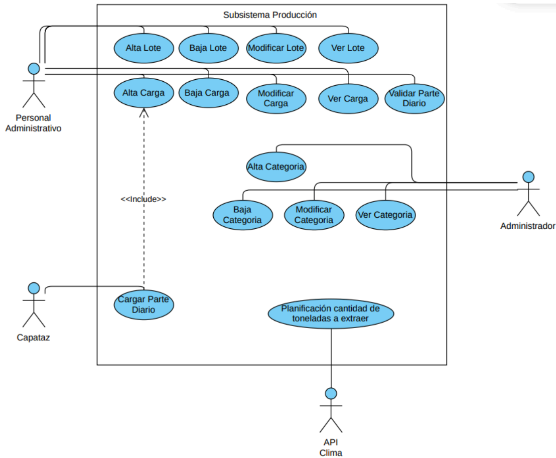
Figura 1 - Diagrama Caso Usos Subsistema Producción
