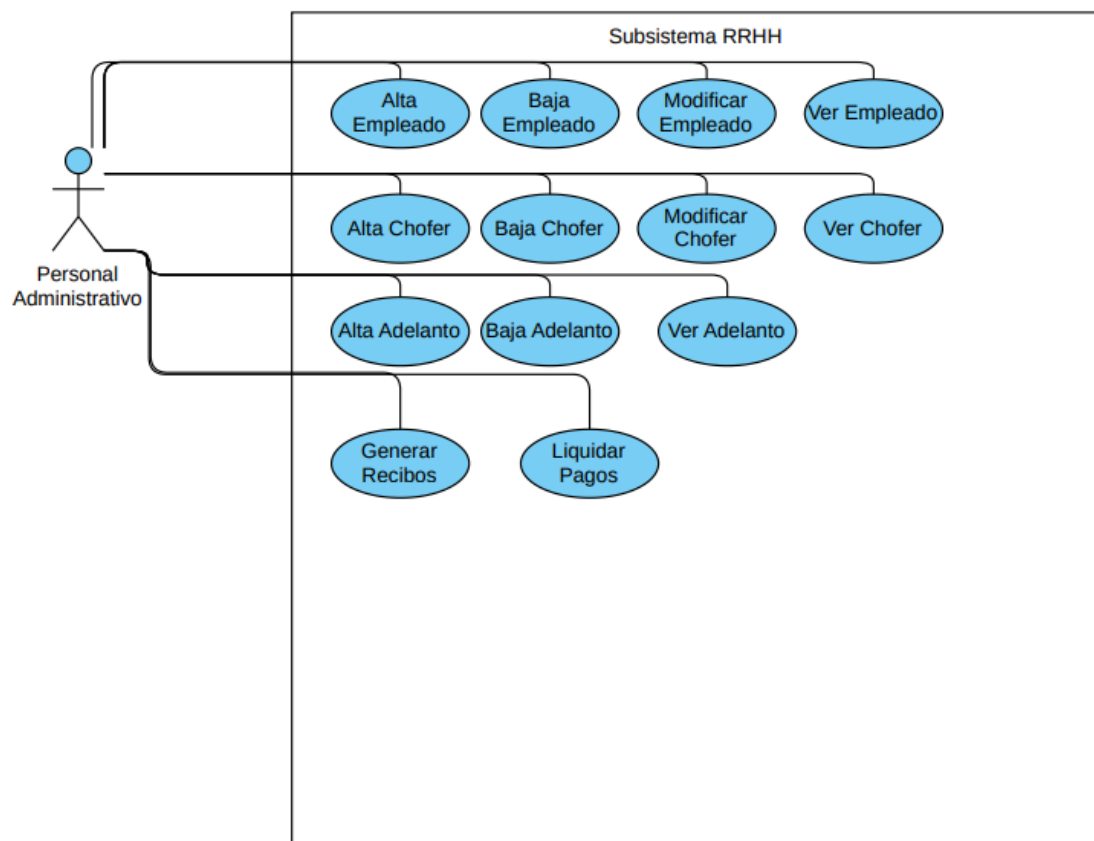
Figura 3 - Diagrama Caso Usos Subsistema Recursos Humanos
